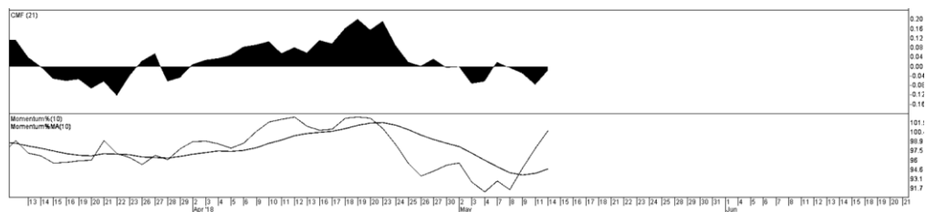
Kinerja IHSG
